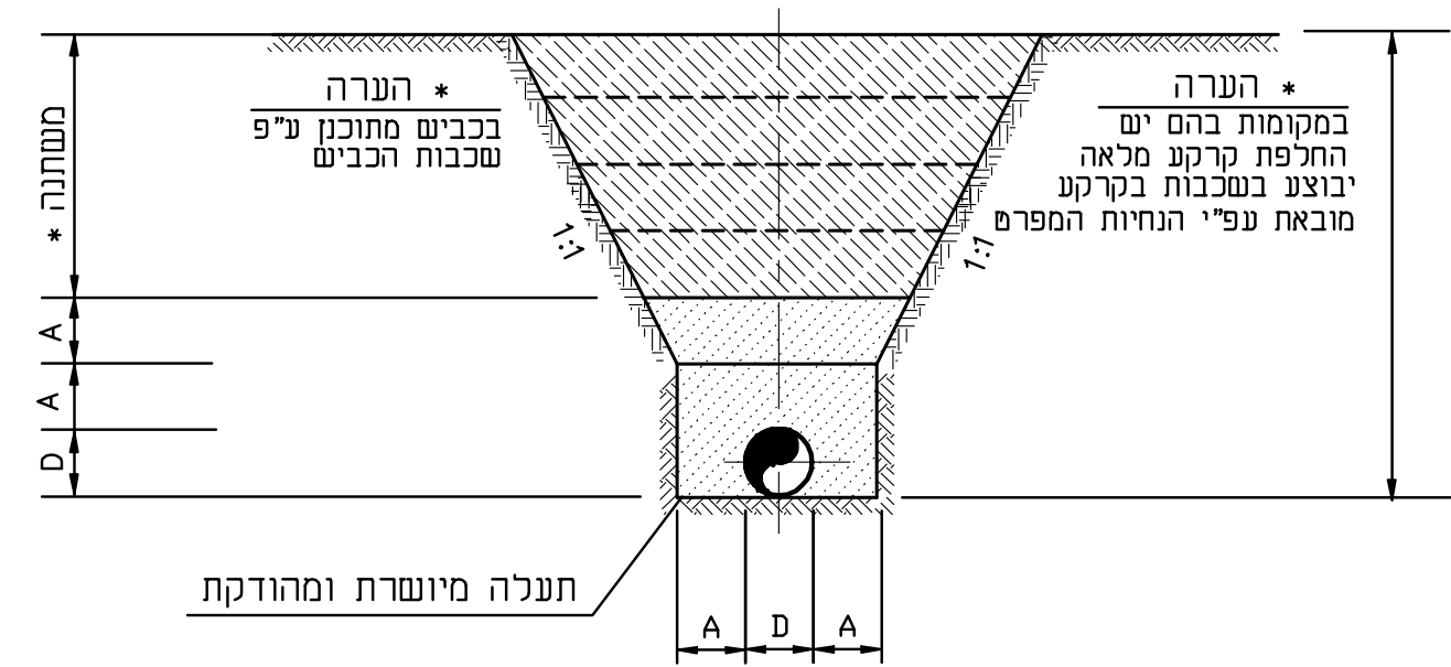
פרט "B" הנחת צנור פלדה עטוף בטון בתעלה ללא מצע
