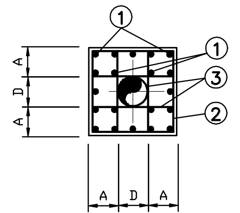
פרט "B" פרט עטיפת בטון סביב צנור
