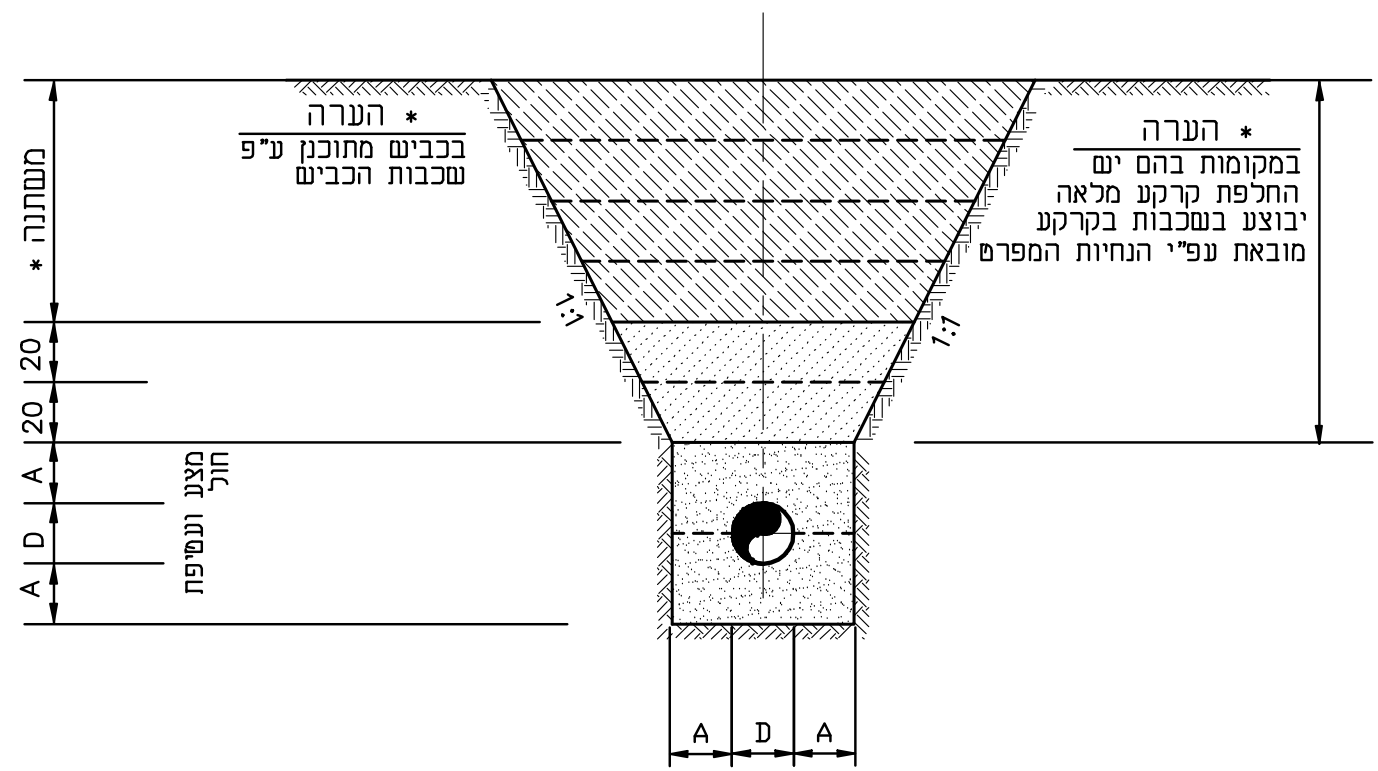
פרט "A" הנחת צנור בתעלה עם מצע
